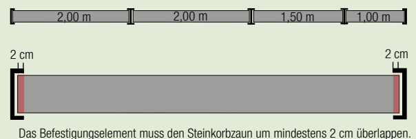
Draufsicht
